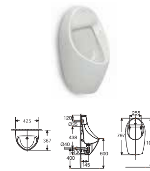
EURET 小便器 (後入水) Z35945F000 $4,590 425 367 797 mm
