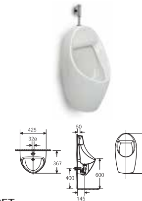
EURET 小便器 (頂入水) Z35945H000 $4,590 425 367 797 mm
