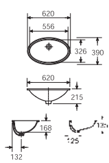
DIVERTA 枱底盆
