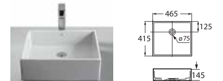
SOFIA 枱上盆
